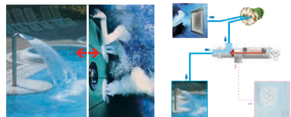
Automatische omschakeling met 2 3-wegventielen tussen 2 waterattracties
